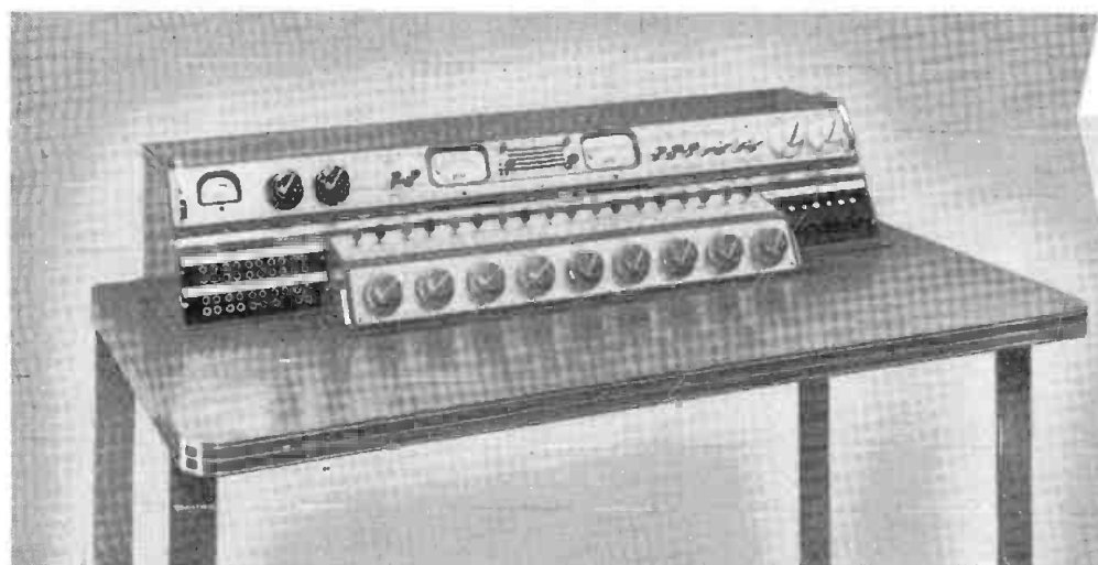
Console...230B
